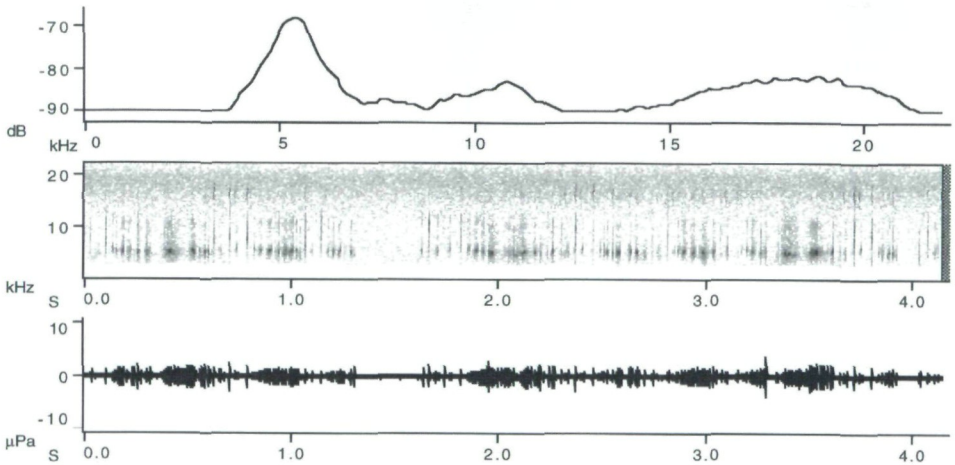
Abb. 3: Rivalengesang Aug 17.5.97. Oszillogramm von zwei Versen.
