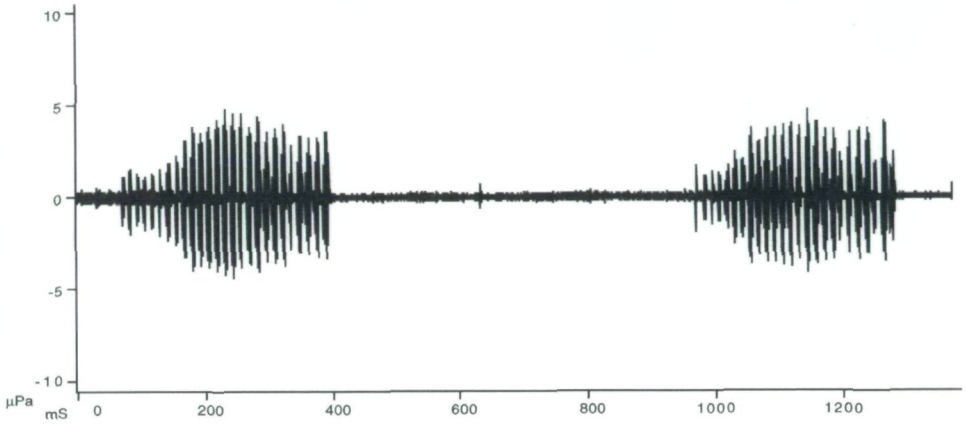
Abb. 3: Rivalengesang Aug 17.5.97. Oszillogramm von zwei Versen.
