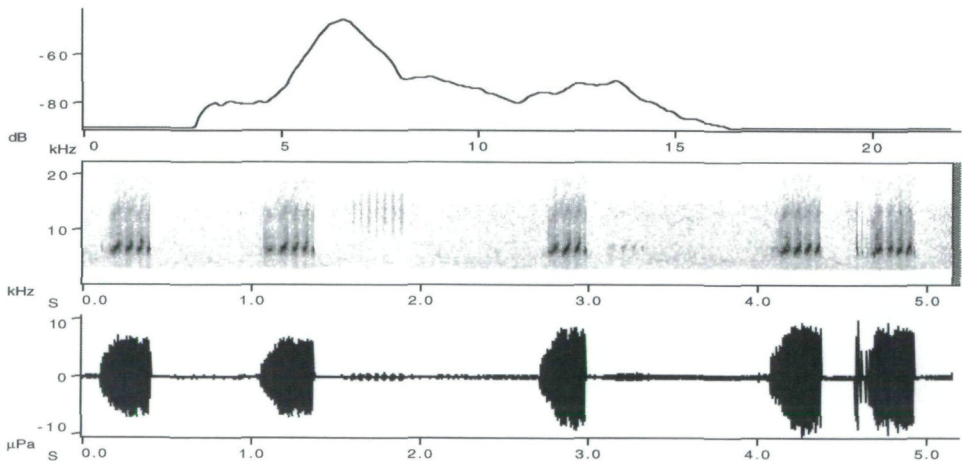
Abb. 1: Rivalengesang Aug 17.5.97. Leistungsspektrum, Sonogramm und Oszillogramm von vier Versen.
