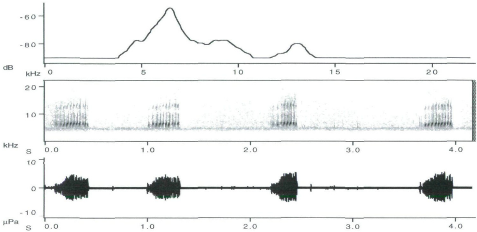
Abb. 1: Rivalengesang Aug 17.5.97. Leistungsspektrum, Sonogramm und Oszillogramm von vier Versen.
