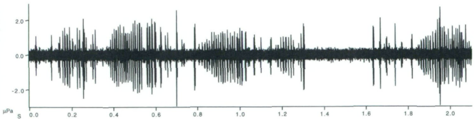
Abb. 5: Werbegesang Aug 15.5.97, Oszillogramm.
